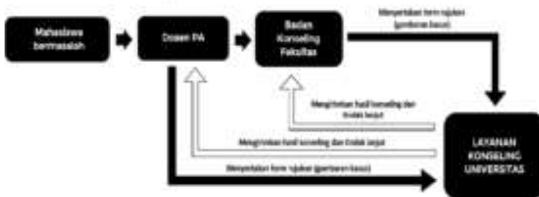
Gambar 17. Alur Rujukan
